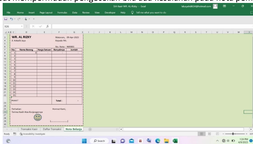
Gambar 3. Nota Pembelian
