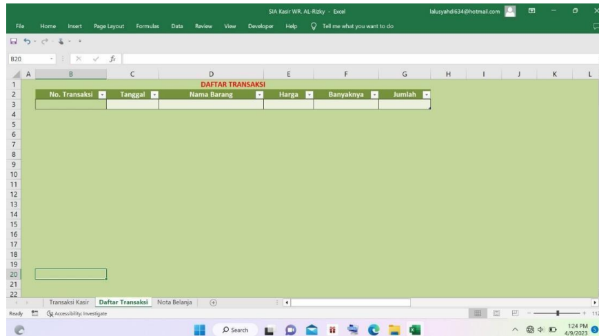
Gambar 2. Daftar Transaksi
