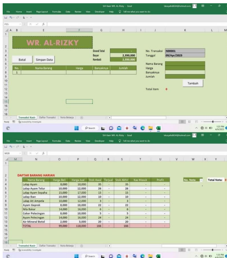
Gambar 1 & 2. Transaksi Kasir
